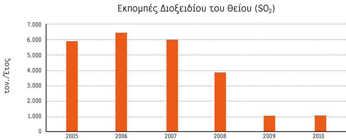
Διάγραμμα 4.4.4: Εκπομπές διοξειδίου του θείου (δουλευτήριο ΟΚΤΑ)
